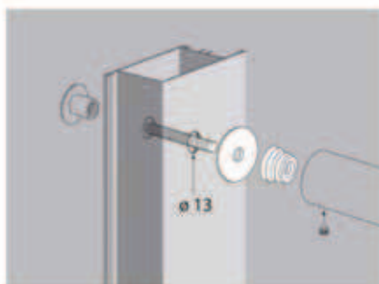
Fissaggio singolo passante per alluminio, legno e PVC.
