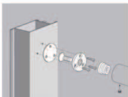
Fissaggio singolo o doppio non passante per alluminio, legno e PVC.
